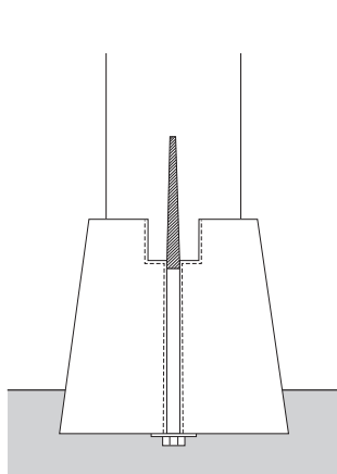
コーチボルト止め工法
