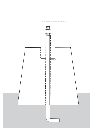
アンカーボルト止め工法
